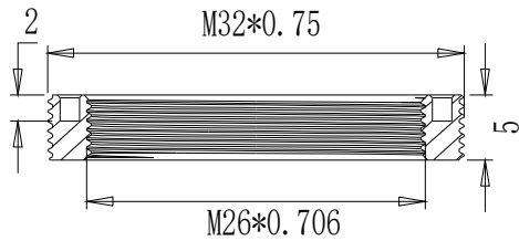
截面 A-A
