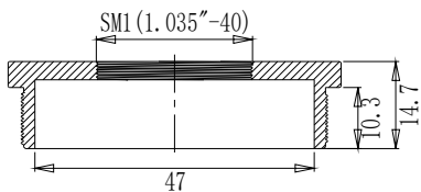
截面 A-A
