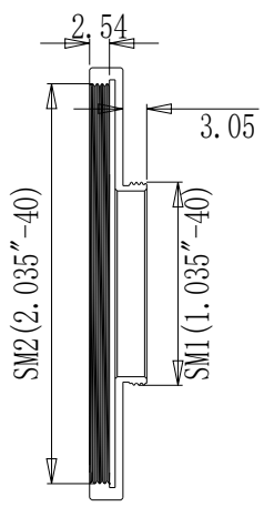
截面 A-A
