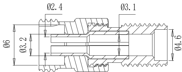
截面 A-A
