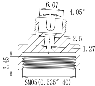
截面 A-A
