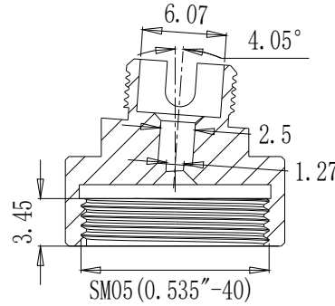
截面 A-A
