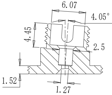
截面 A-A
