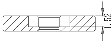
截面 A-A
