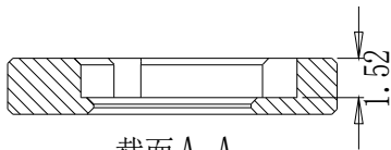
截面 A-A
