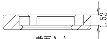
截面 A-A
