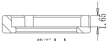
截面 A-A
