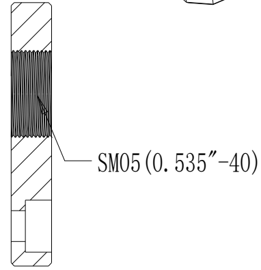
截面 A-A
