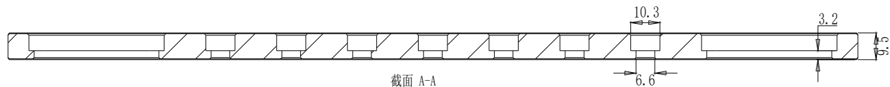
截面 A-A
