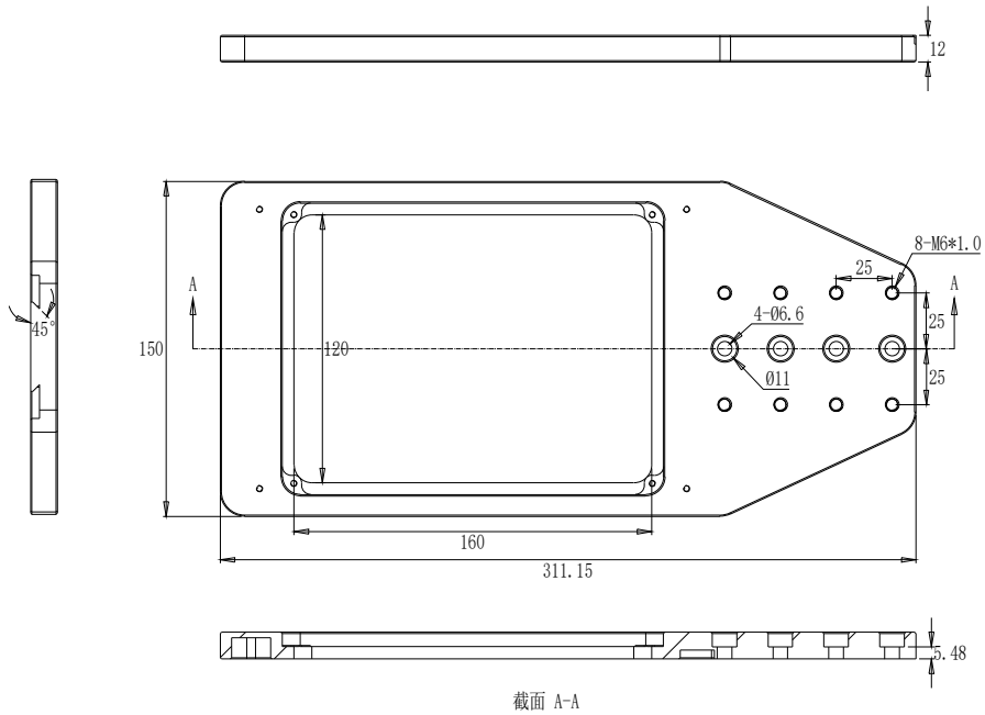
截面 A-A
