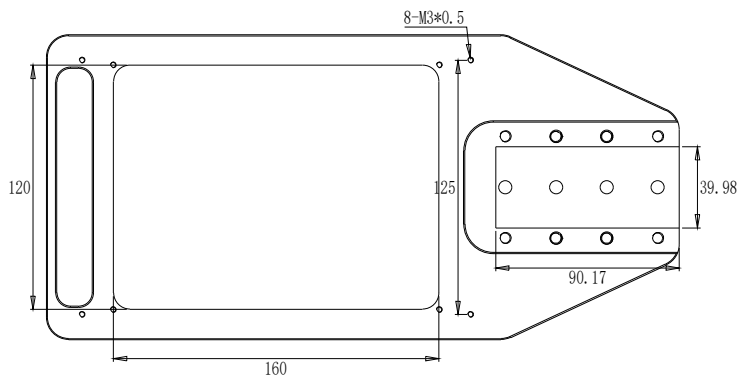
截面 A-A
