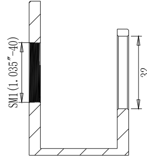
截面 A-A
