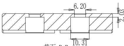
截面 B-B
